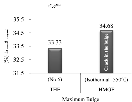
شکل ۳۴ نسبت انبساط لوله دولایه در فرآیندهای شکل‌دهی (THF) و (HMGF)
