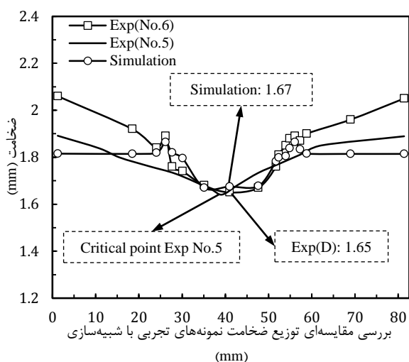
شکل ۳۱ بررسی مقایسه‌ای توزیع ضخامت نمونه‌های تجربی با شبیه‌سازی در فرآیند هیدروفورمینگ
