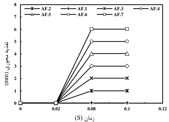
شکل ۲۸ الگوی تغذیه محوری مرحله‌ای در شکل‌دهی لوله‌های دولایه
