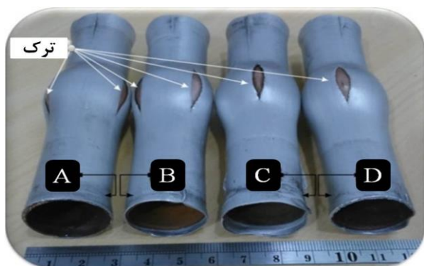
شکل ۱۵ نمونه‌های دولایه شکل داده شده در فرآیند HMGF (A) هم‌دما 550 درجه سانتی‌گراد، (B) گرادیانی 550 درجه سانتی‌گراد، (C) گرادیانی 570 درجه سانتی‌گراد، (D) هم‌دما 570 درجه سانتی‌گراد
