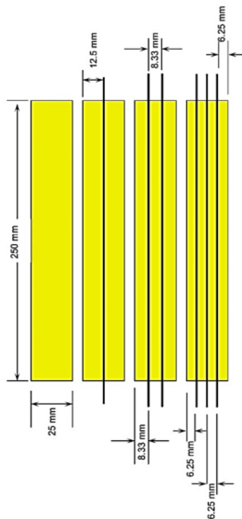
Fig. 6 Geometrical properties of cotton/epoxy laminated composite specimens with or without NiTi wires. شکل 6 مشخصات هندسی نمونه‌های کامپوزیت لایه‌ای پنبه/لاتکس با یا بدون سیم‌های نیتینول
