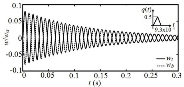
شکل ۱۰ خیز دینامیکی نقطه میانی رویه بالا و پایین تیر ساندویچی با هسته انعطاف‌پذیر جانی تحت بار ضربه با شرایط هندسی h_c/h=0.94 و L/h=10
