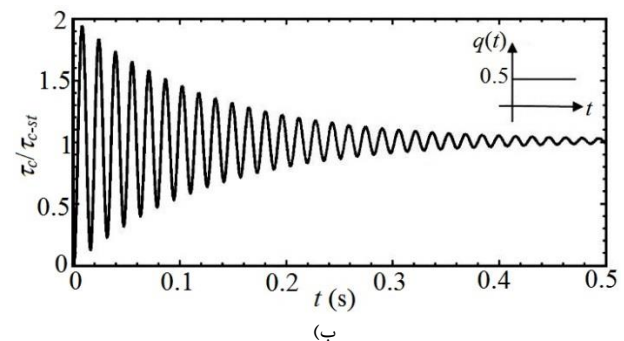
شکل ۱۶ خیز دینامیکی (ب) تنش برشی هسته‌ی تیر ساندویچی با دو سر تکیه‌گاه ساده تحت بارگذاری پله طبق مدل GHM
