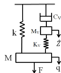
شکل ۴ مدل مکانیکی روش GHM [۱۴]
