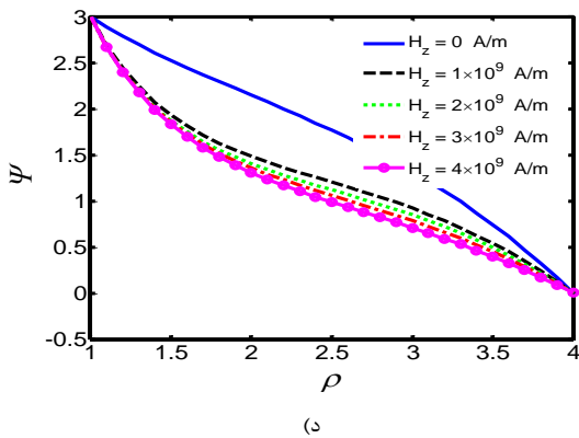
شکل ۹ الف) کرنش (ب) تنش (ج) جابه‌جایی شعاعی (د) توزیع پتانسیل الکتریکی برحسب پارامتر \rho به ازای مقادیر مختلف H_z و \beta = -1.5, T_i = 10^\circ\text{C}, \Omega = 1
