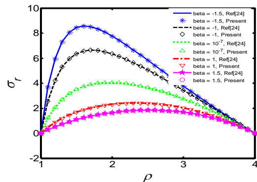
شکل ۵ مقایسه توزیع تنش شعاعی با مرجع [۲۴] برحسب پارامتر بی بعد \rho و پارامتر ناهمگنی \beta و \Omega = 1, H_z = 0, T_0 = 0
