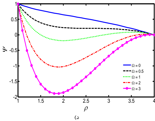
شکل ۴ (الف) کرنش (ب) تنش (ج) جابه‌جایی شعاعی (د) توزیع پتانسیل الکتریکی برحسب پارامتر بعد \rho به ازای مقادیر \Omega و H_z = 1 \times 10^9 A/m و \beta = -1.5, T_0 = 50^\circ C
