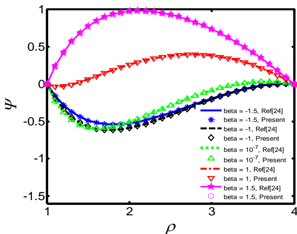
شکل ۲ مقایسه توزیع پتانسیل الکتریکی با مرجع [۲۴] برحسب پارامتر بی بعد \rho و پارامتر نا همگنی \beta و \Omega = 1 ، H_z = 0 ، T_0 = 0
