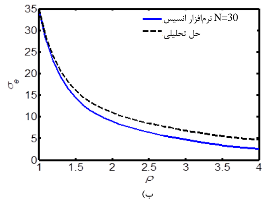
شکل ۱۳ مقایسه نتایج تحلیلی با نتایج عددی با استفاده از نرم افزار انسیس به ازای T_0 = 100, H_z = 0, \beta = -1, \Omega = 1 کرنش (ب) تنش
