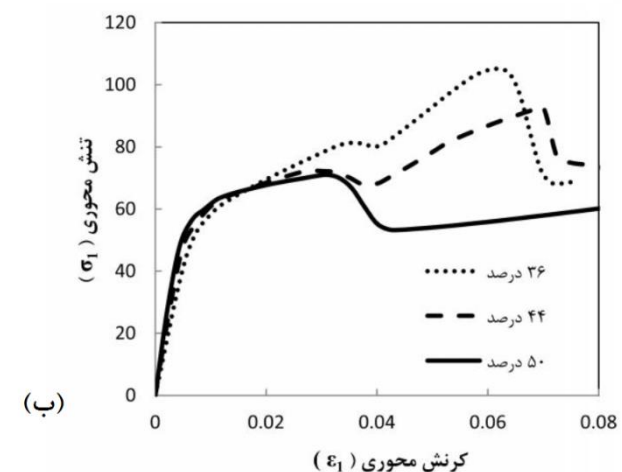
شکل ۱۸ نمودار تنش- کرنش در المان‌های حجمی با یک لیف و در حضور هر دو نوع خرابی جدایش الیاف/ ماتریس و ترک ماتریسی و به ازای (الف) شعاع‌های مختلف الیاف با درصد حجمی ثابت ۵۰٪، (ب) درصدهای حجمی مختلف الیاف و شعاع یکسان ۴.۵ میکرومتر
