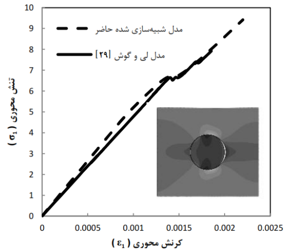
شکل ۷ مقایسه نتایج تنش و کرنش مدل حاضر در صحت‌سنجی با مدل لی و گوش [۲۹].
