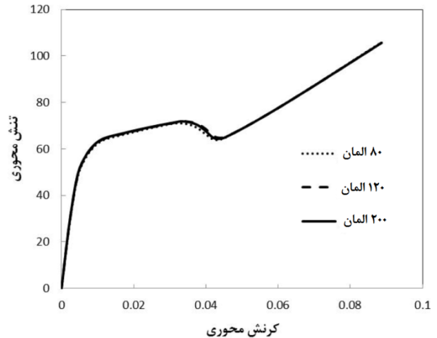
شکل ۱۱ آنالیز حساسیت مش
