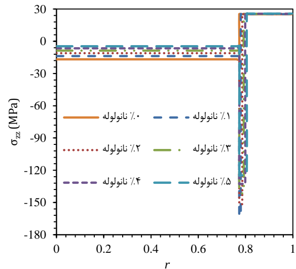
شکل ۵ توزیع تنش طولی در سلول واحد در حالت موازی بودن رشته کربنی و نانولوله
