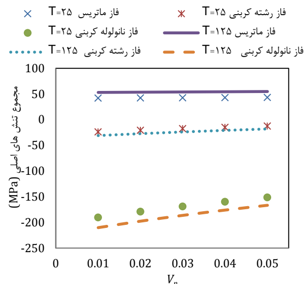
شکل ۱۳ مقایسه مجموع تنش‌های اصلی به دست آمده در دماهای متفاوت محیط و دمای پخت
