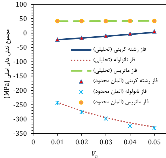
شکل ۱۲ مقایسه مجموع تنش‌های اصلی روش المان محدود و روش تحلیلی در حالت قرارگرفتن نانولوله به صورت حلقه‌گون بر رشته کربنی
