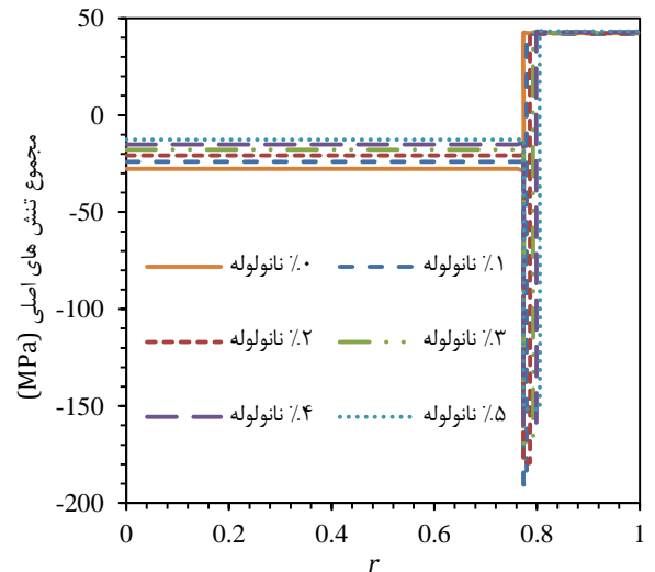
شکل ۶ توزیع مجموع تنش‌های اصلی در سلول واحد در حالت موازی بودن رشته کربنی و نانولوله
