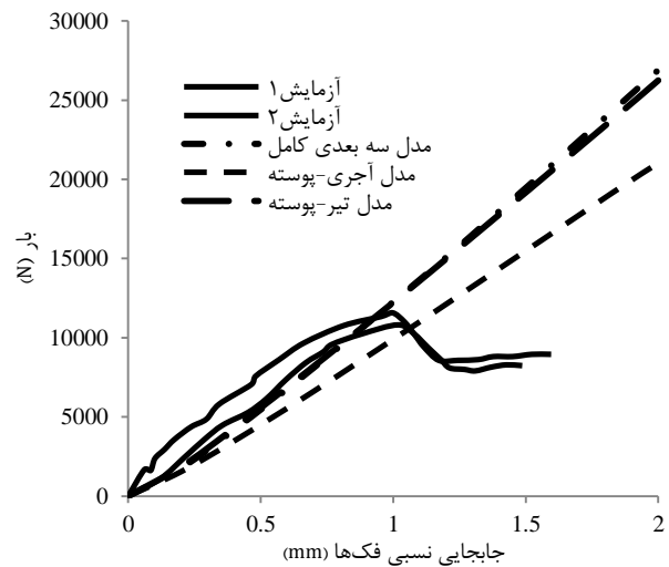
شکل ۷ مقایسه نتایج تحلیل المان محدود صورت گرفته با مدل‌های آجری-آجری؛ پوسته-آجری، پوسته-میله‌ای و دو تست تجربی
