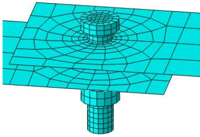
شکل ۲ مدل آجری-پوسته
