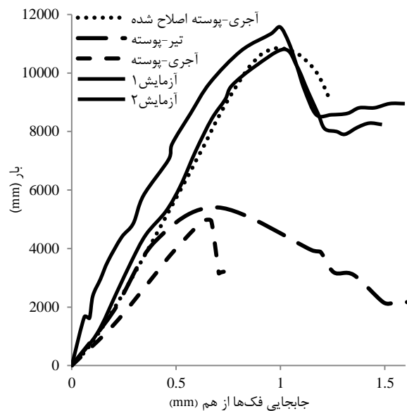
شکل ۹ مقایسه نتایج مدل‌های المان محدود مختلف اتصال پیچی با در نظر گرفتن معیار هاشین جزء کامپوزیتی و ناحیه پلاستیک پیچ و جزء اتصال آلومینیومی
