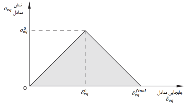
شکل ۴ منحنی تنش معادل-جاب‌جایی معادل
