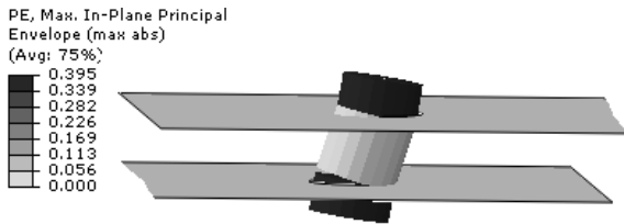
شکل ۱۰ حداکثر کرنش پلاستیک معادل در جابه‌جایی ۲ میلی‌متر (مدل تیر-پوسته)
