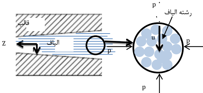
شکل ۱ شماتیک حرکت الیاف و نحوه نفوذ پلیمر
