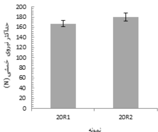
شکل ۲۲ مقایسه نمونه‌های ۲۰R۱ و ۲۰R۲ از نظر حداکثر نیروی خمشی
