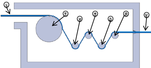
شکل ۳ شماتیک قالب استفاده شده (۱: الیاف ورودی، ۲: ۵، ۴، ۳، ۲ و ۶: پین‌ها، ۷: محصول خروجی)
