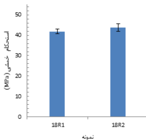
شکل ۲۱ مقایسه نمونه‌های ۱۸R۱ و ۱۸R۲ از نظر استحکام خمشی
