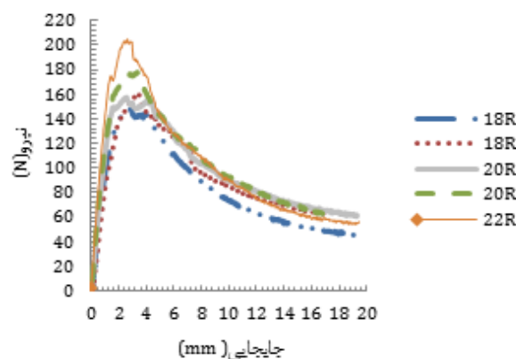
شکل ۱۷ نمودار نیرو-جابجایی نمونه‌های مورد آزمایش
