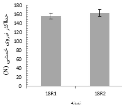
شکل ۲۰ مقایسه نمونه‌های ۱۸R۱ و ۱۸R۲ از نظر حداکثر نیروی خمشی
