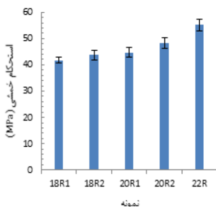
شکل ۱۹ نمودار مربوط به استحکام خمشی
