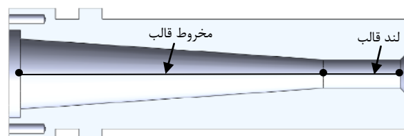
شکل ۷ بخش مادگی قالب [۲۱]
