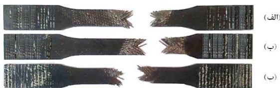
شکل ۷ نمونه‌های کامپوزیتی با بافت اطلسی پس از آزمایش در سه دمای (الف) ۱۰۰، (ب) ۱۵۰، (پ) ۲۰۰ درجه سانتیگراد
